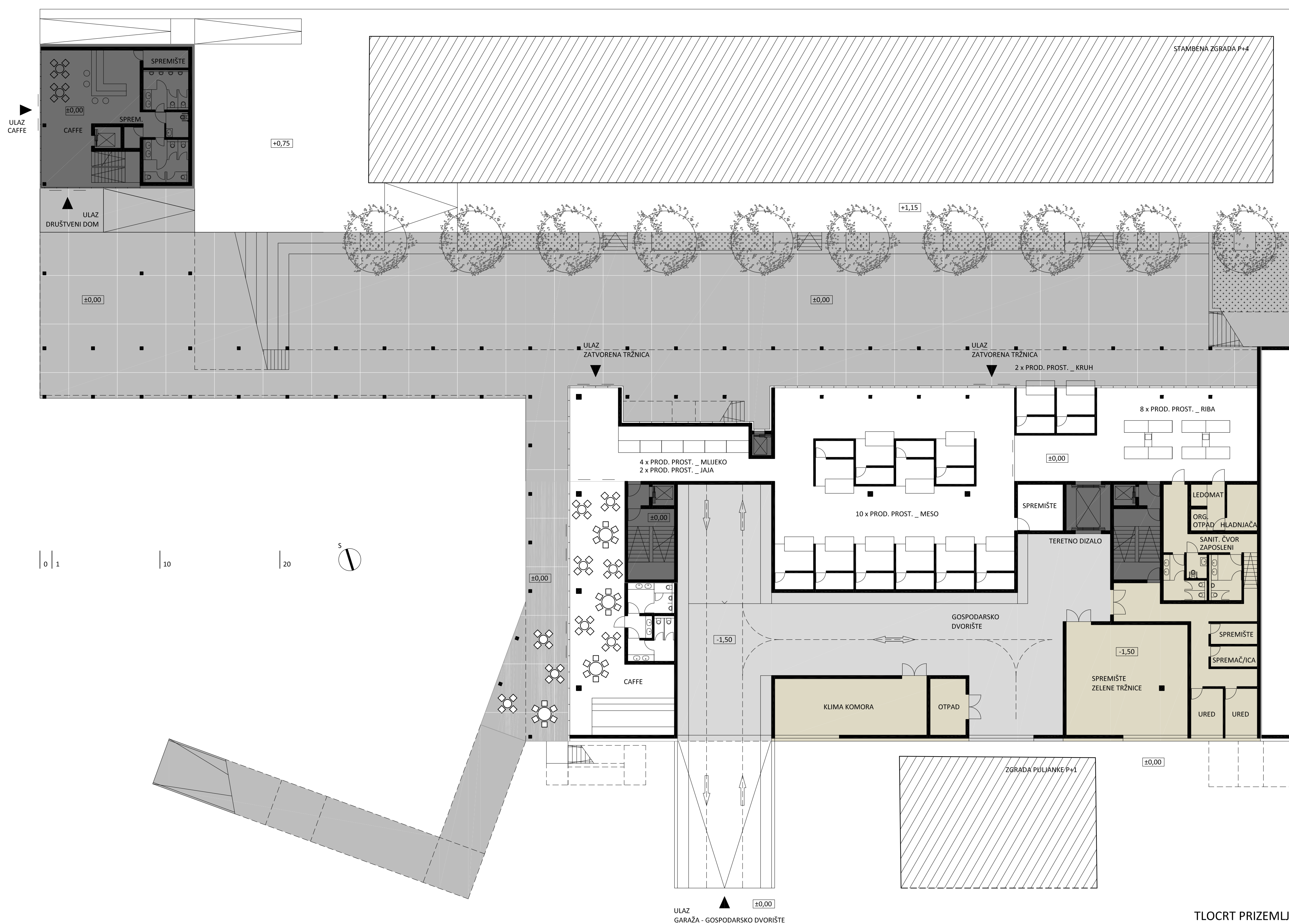
TLOCRT PRIZEMLJA
