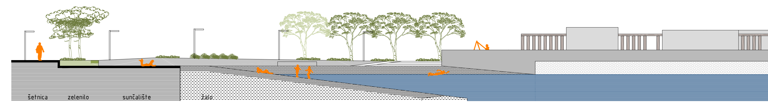
presjek_plaža_mj 1:200
