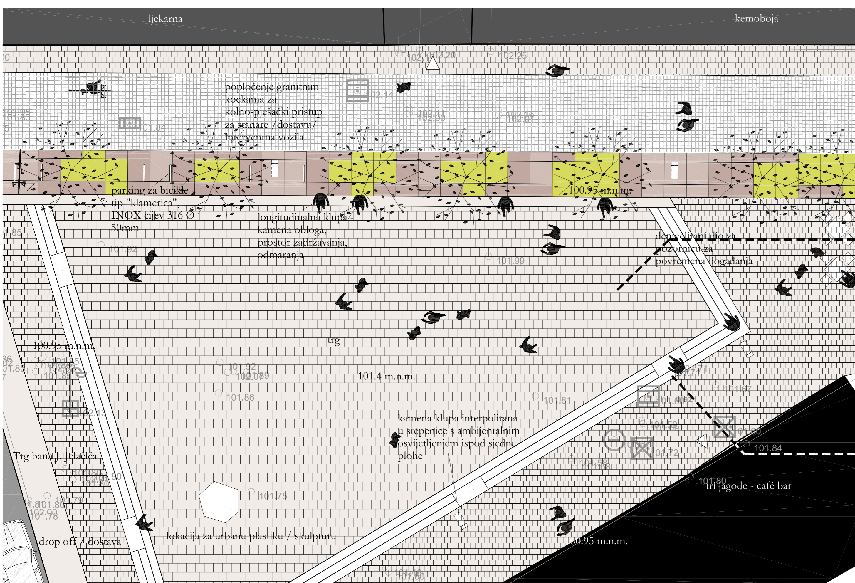
Detalj dijela Ulice S. S. Kranjčevića kod spoja s Trgom bana Josipa Jelčića mj 1:100 10 11m 12 15m L sj
