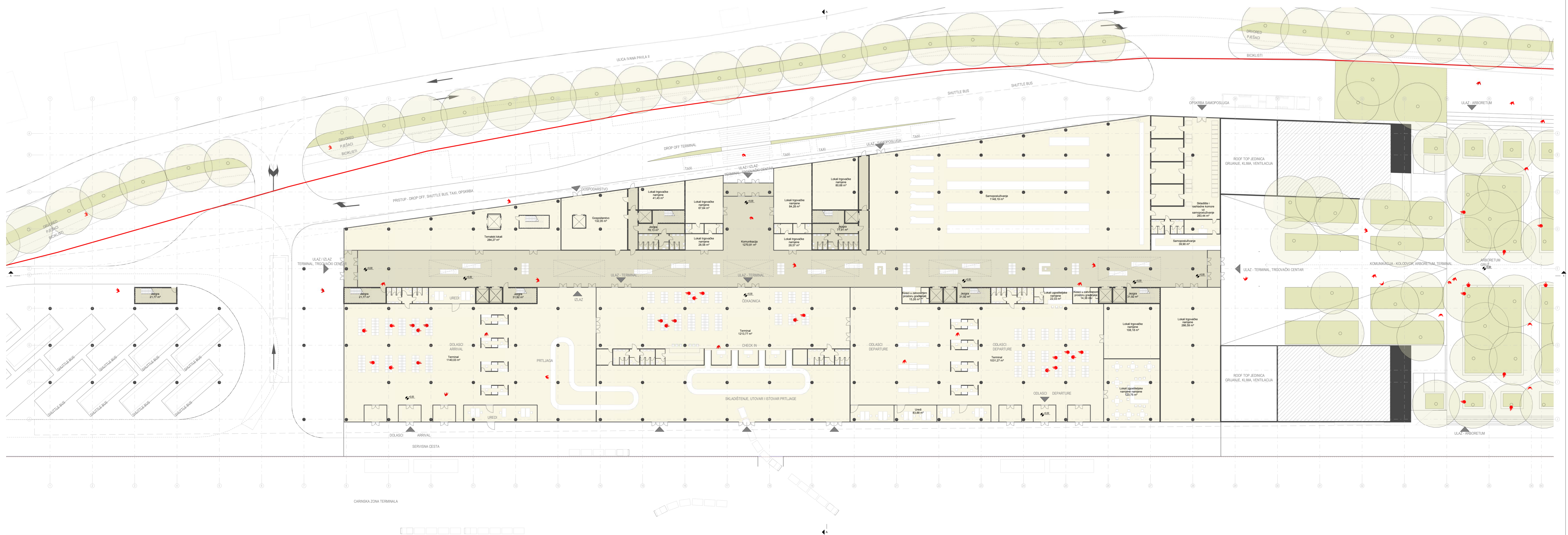
TLOCRT PRIZEMLJA M 1:250
