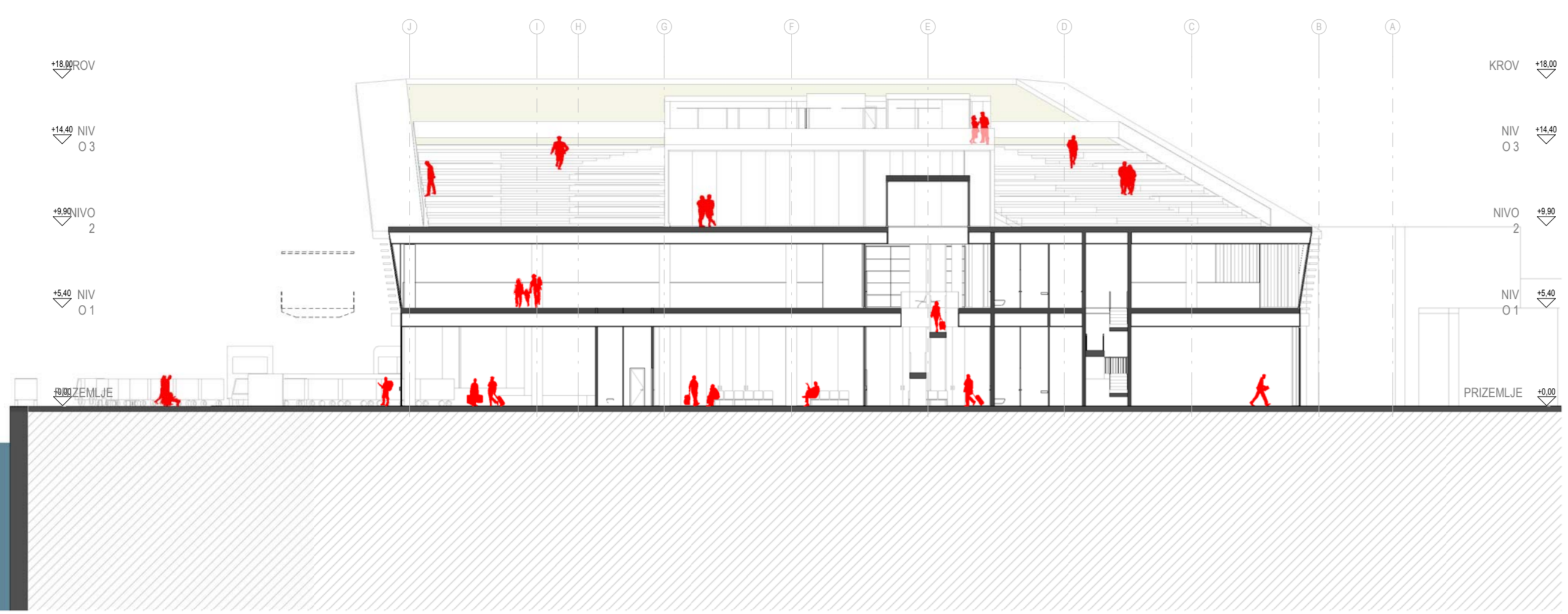
A-A POPREČNI PRESJEK KROZ TERMINAL M 1:250
