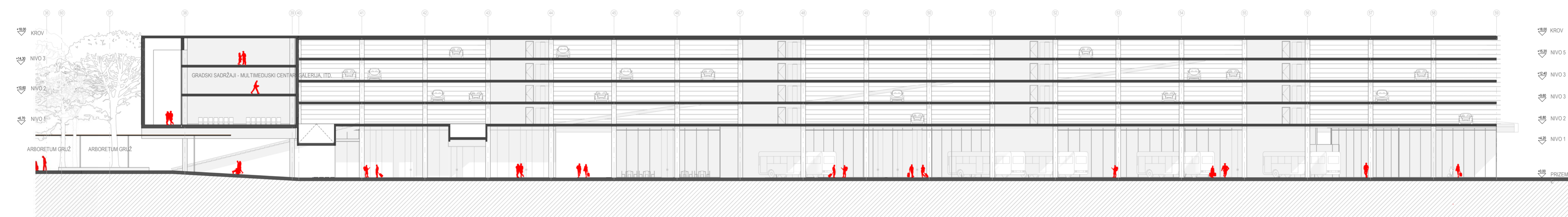
2-2 UZDUŽNI PRESJEK KROZ KOLODVOR I GARAŽNI OBJEKT M 1:250
