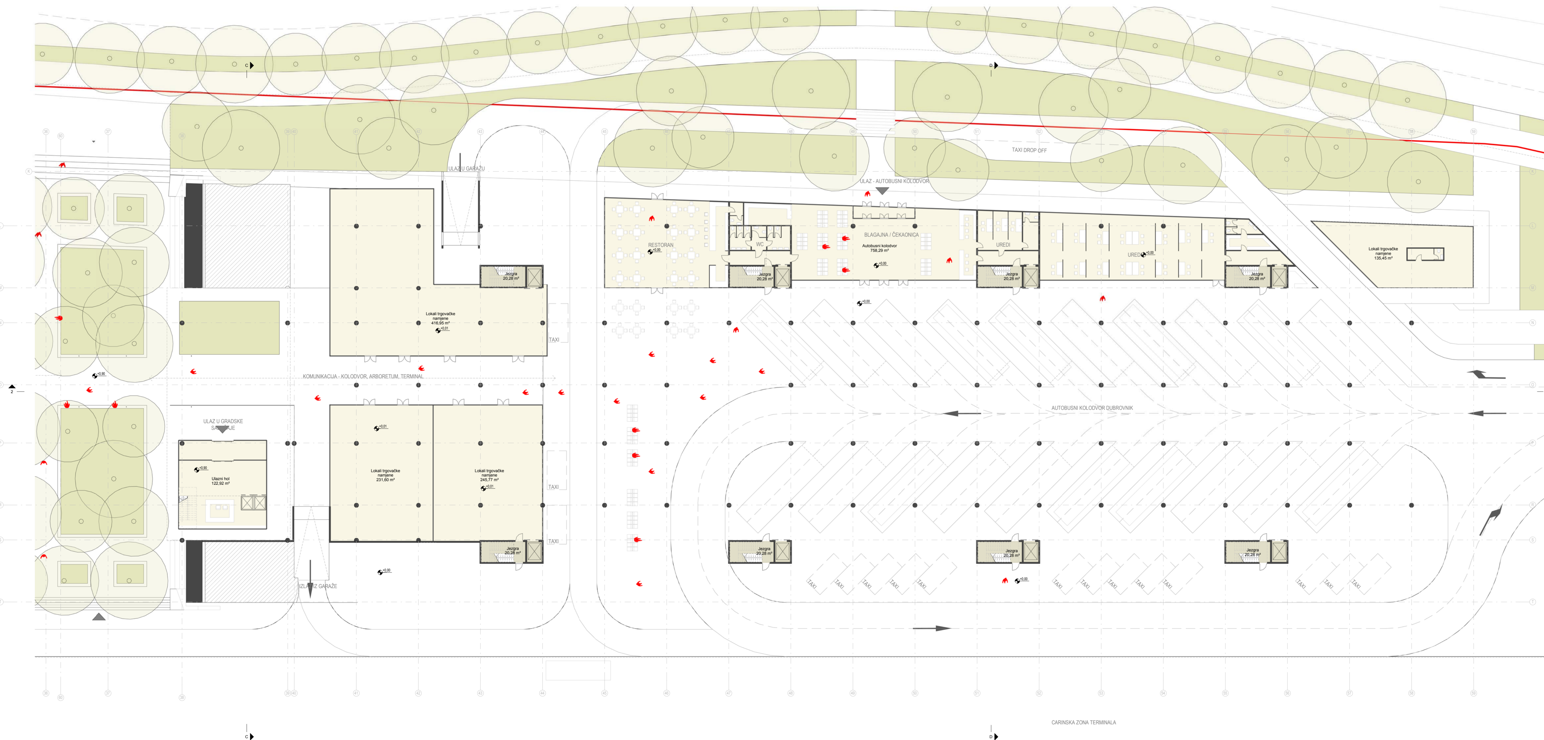
TLOCRT AUTOBUSNOG KOLODVORA M 1:250
