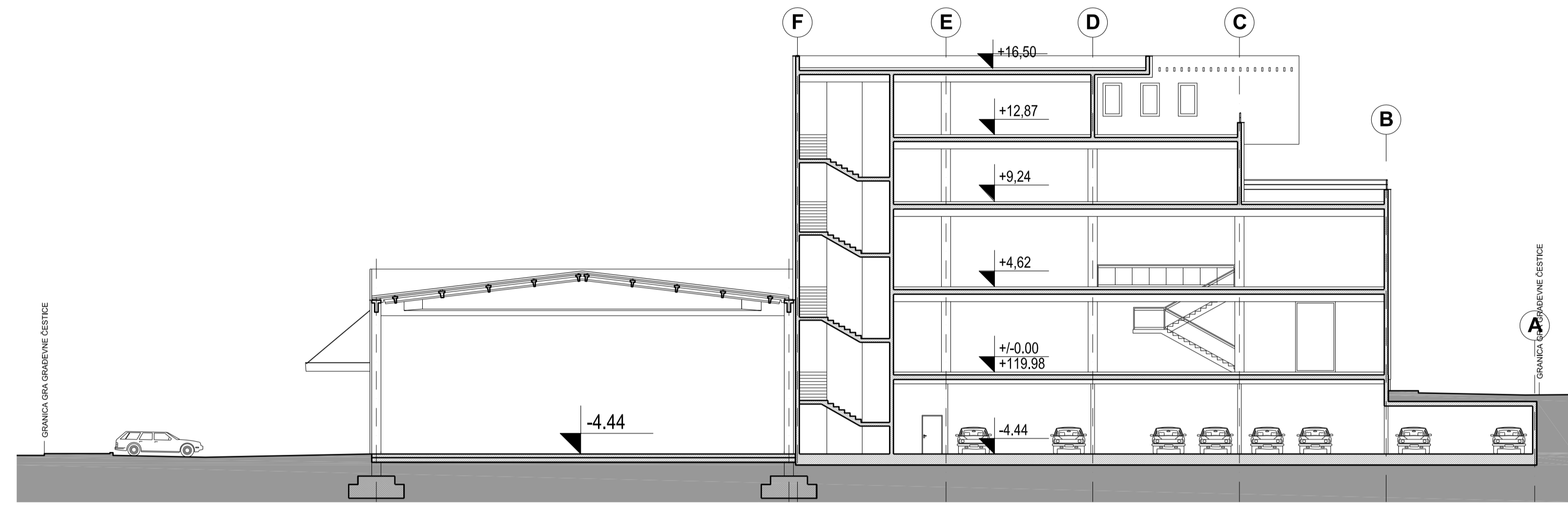
Presjek 1-1
