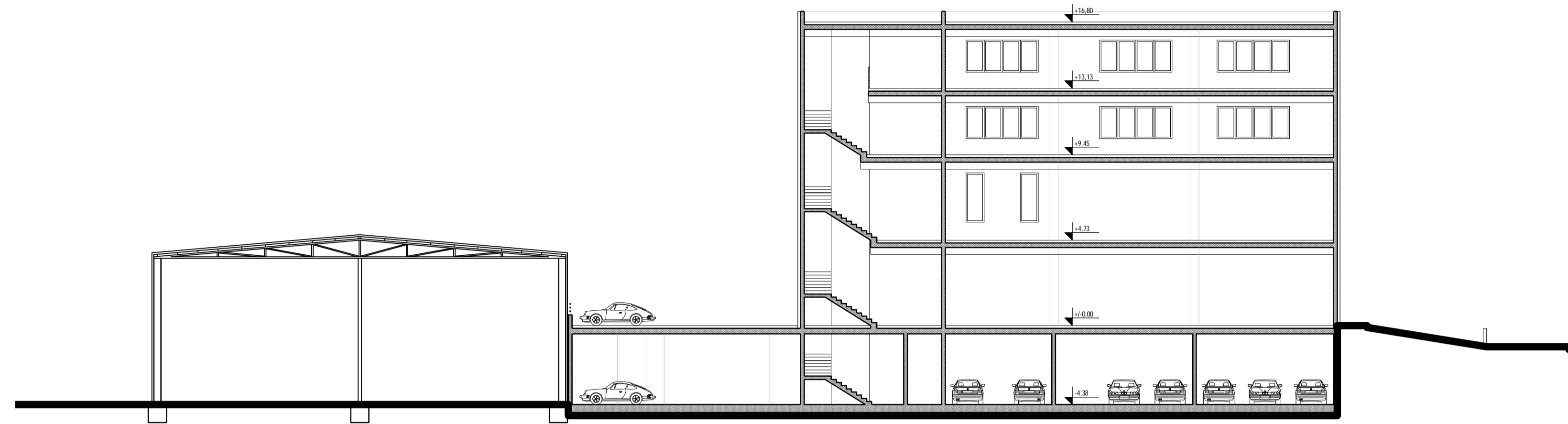
PRESJEK AA
