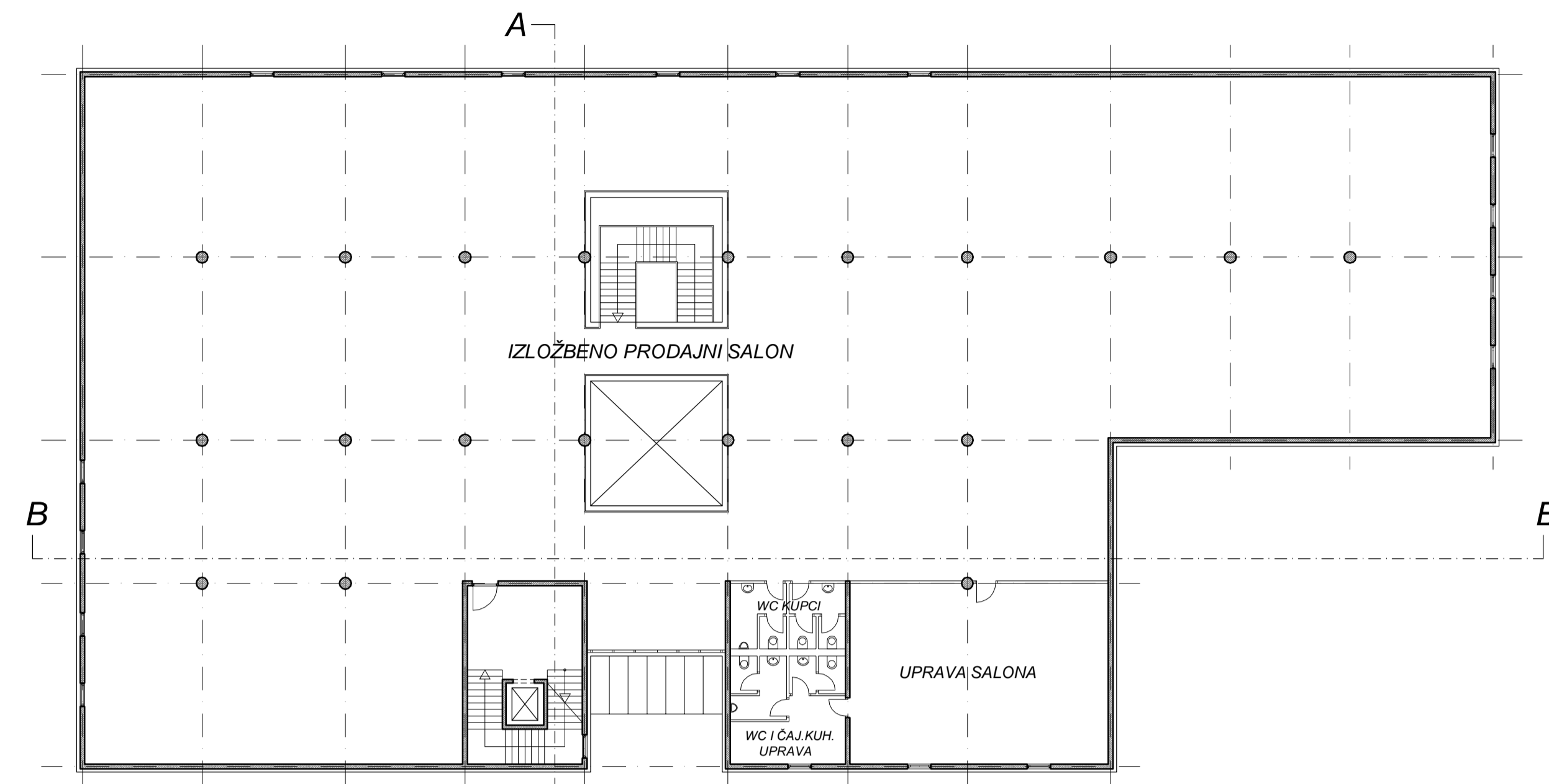
1. KAT
