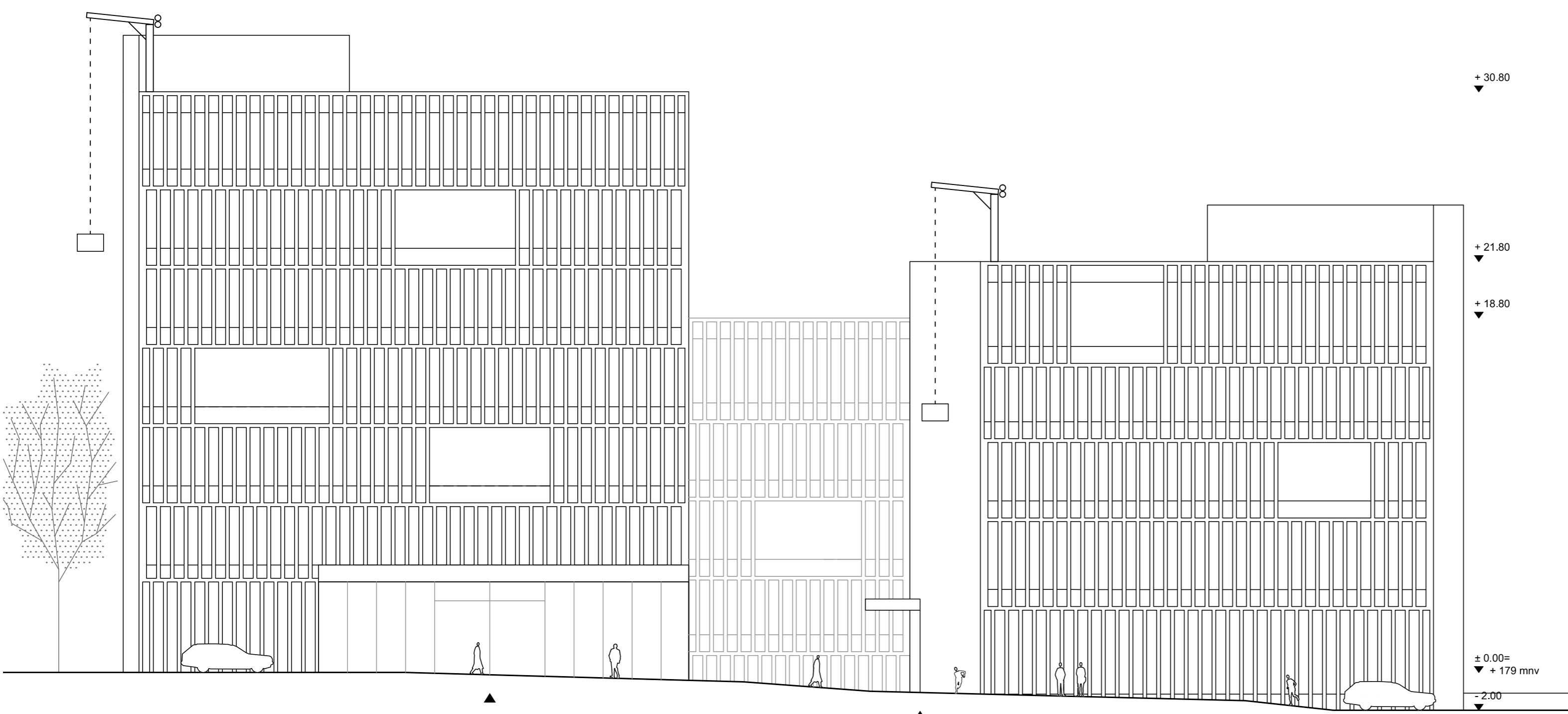
SJEVERNO PROČELJE 1:200
