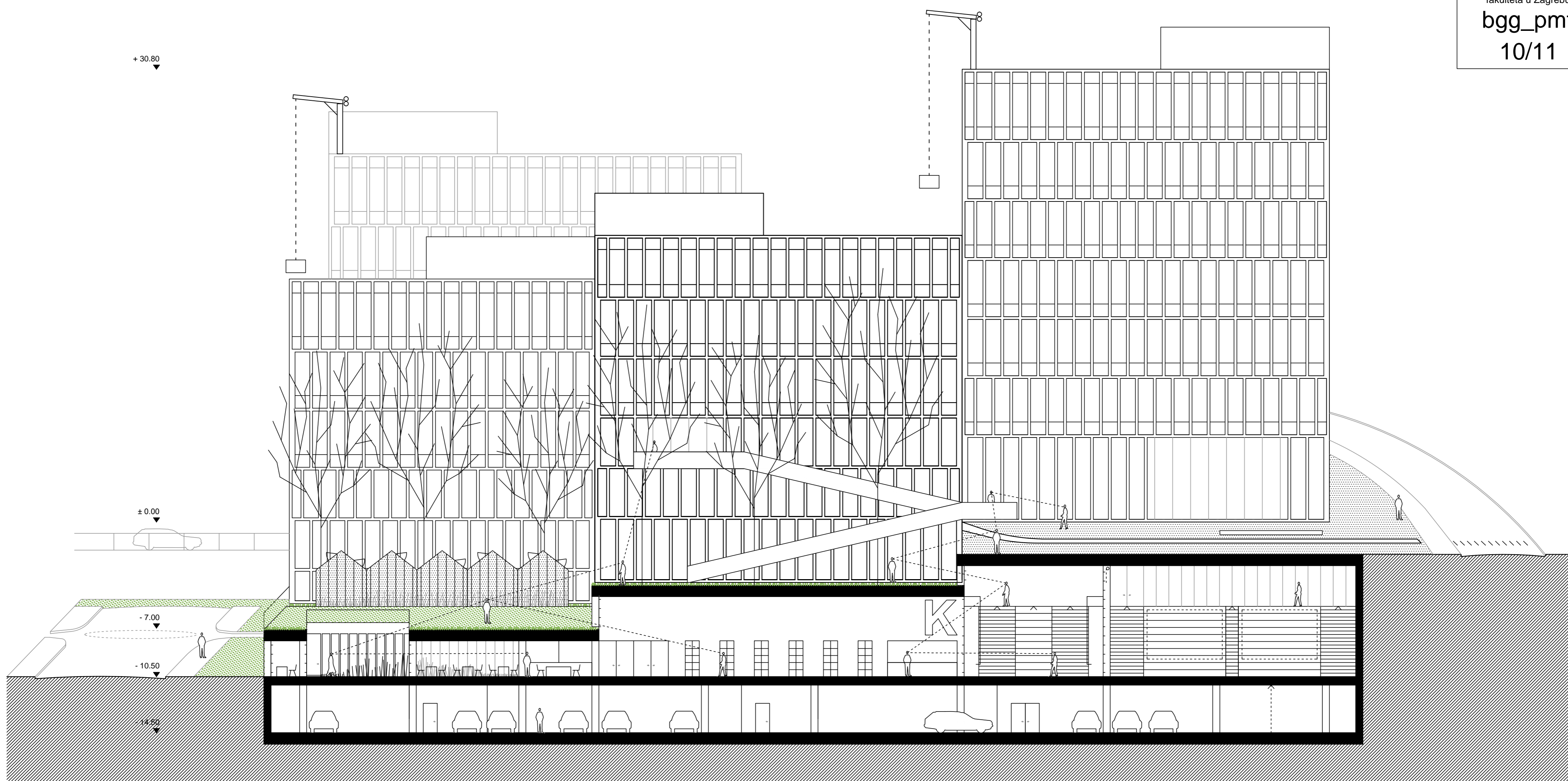
SJEVERNO PROČELJE 1:200
