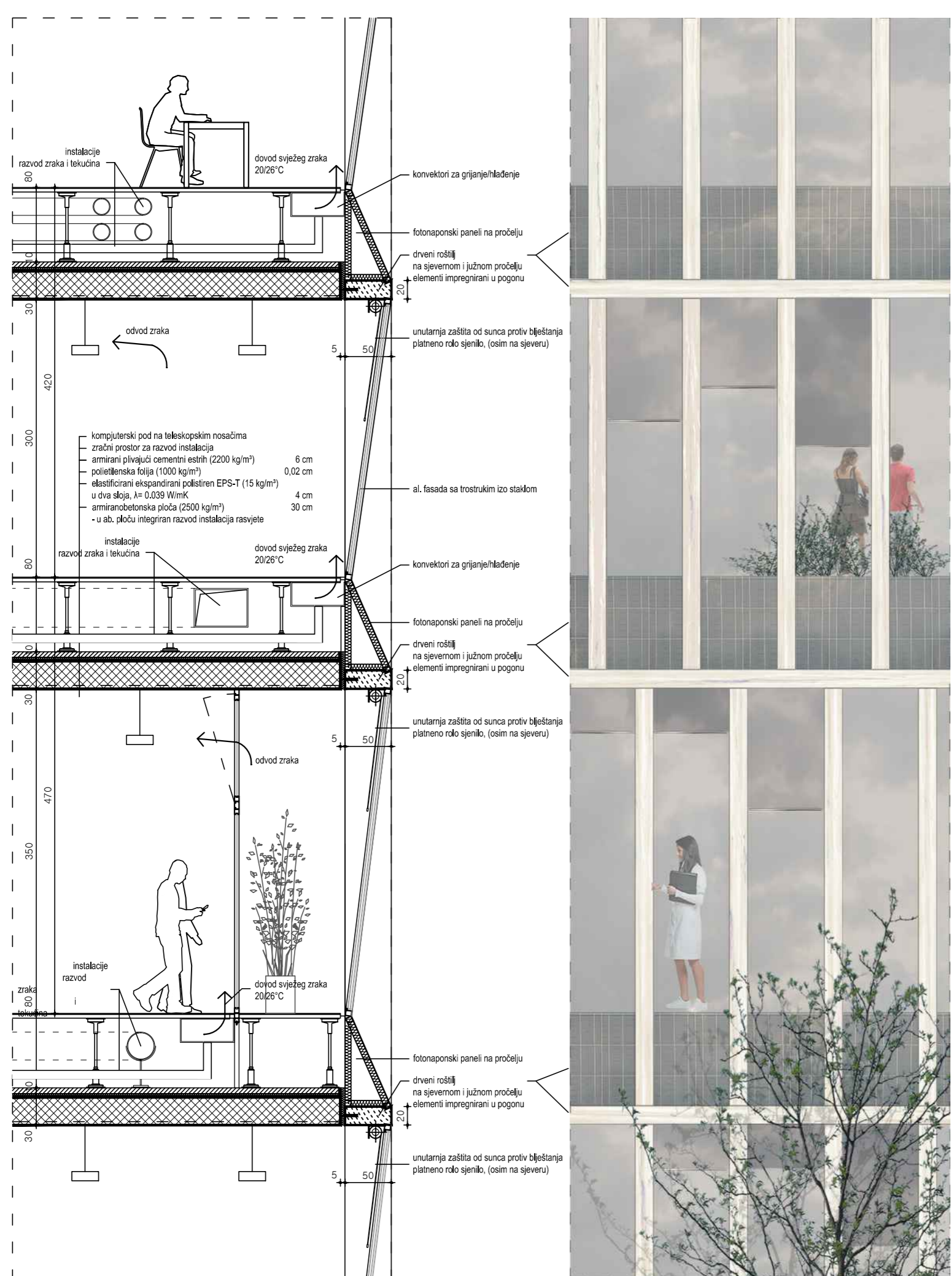
DETALJ PROČELJA 1:50
