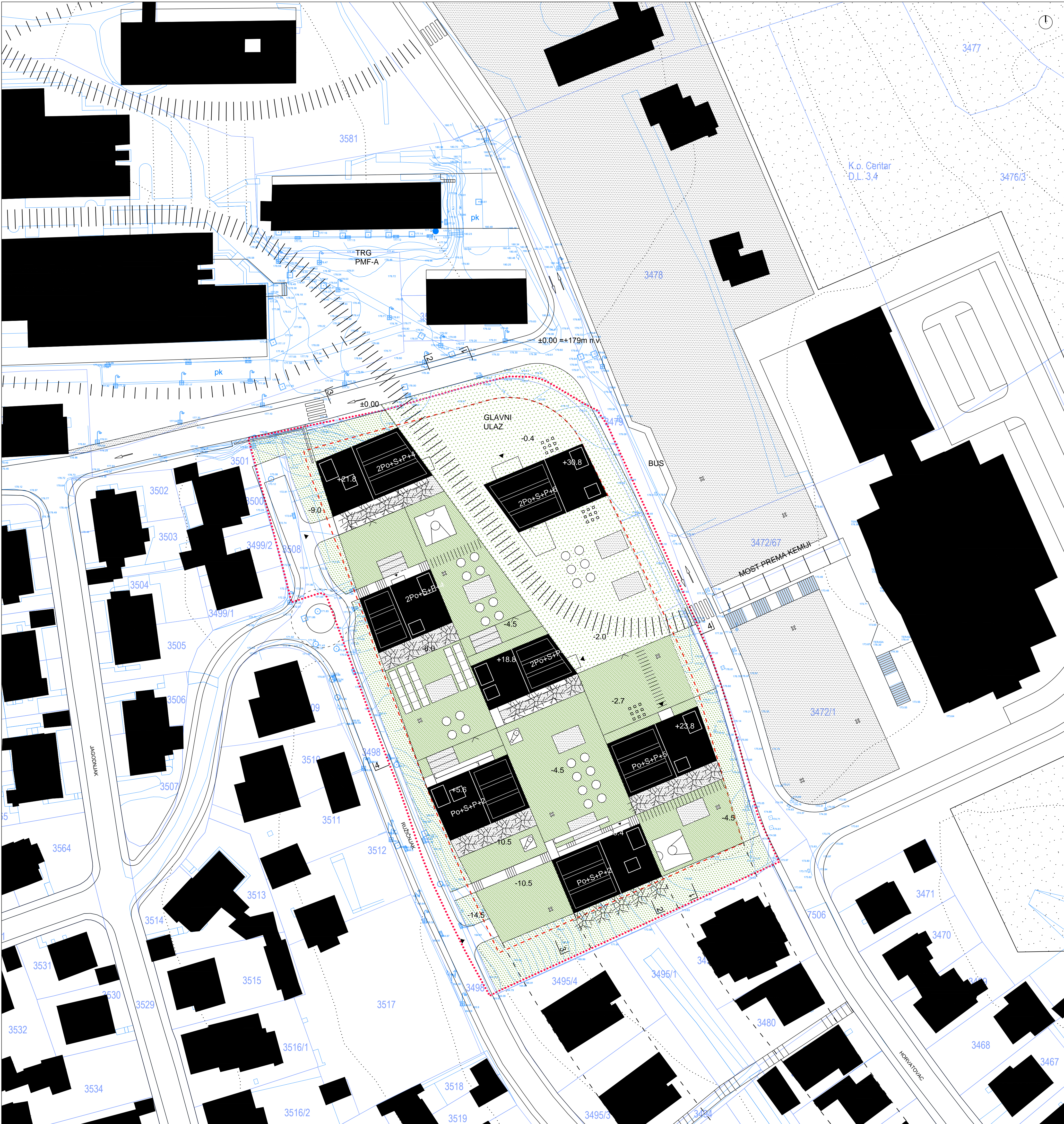
UŽA SITUACIJA 1:500
